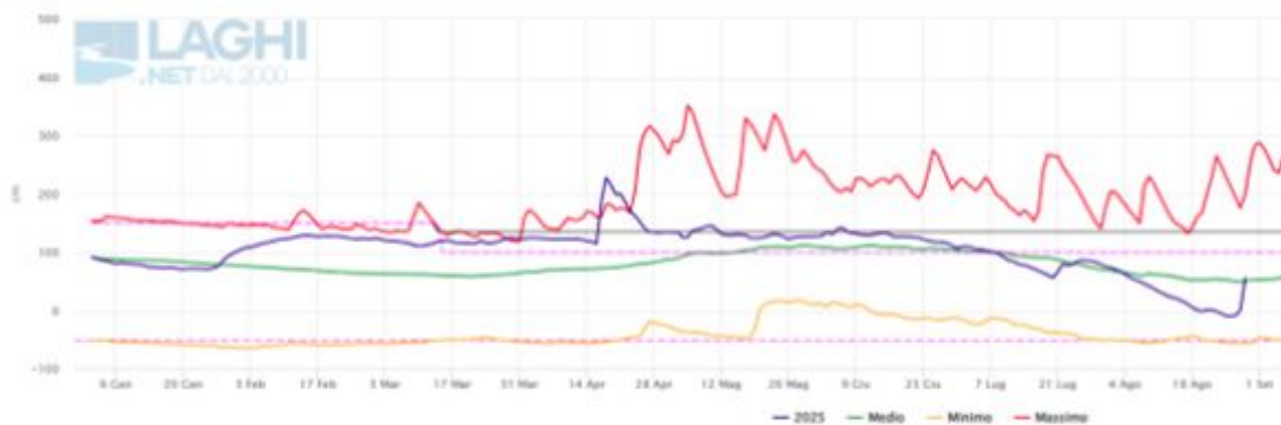
Lago Maggiore – Sesto Calende – Altezze idrometriche ore 8:00 (valori storici relativi al periodo 1942-2023)
